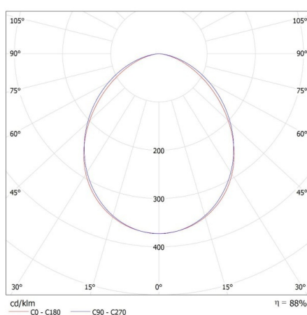
KANLUX S.A. (kat 33886) IQ-LED FL-20W-NW-SE / LDC (Polar)
